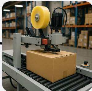
● Kartonierer
