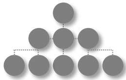
Hierarchische Linienorganisation
