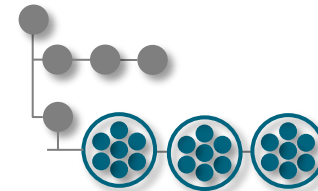
Eingebettete Teamorganisation
