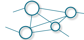
Selbstorganisierte Netzwerkorganisation
