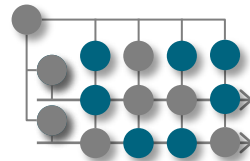
Mehrdimensionale Matrixorganisation
